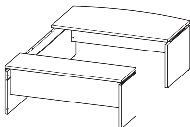
180 × 292 × H 73,5
